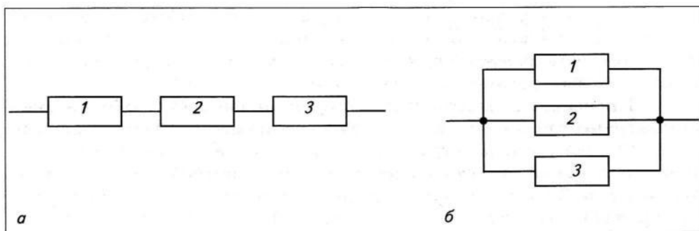
Рис. 56. Соединение проводников:
